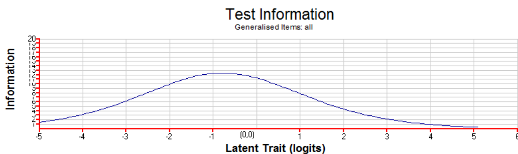
Figura 4.9: Informazione totale sulla prova di Italiano – II sec. II gr.
