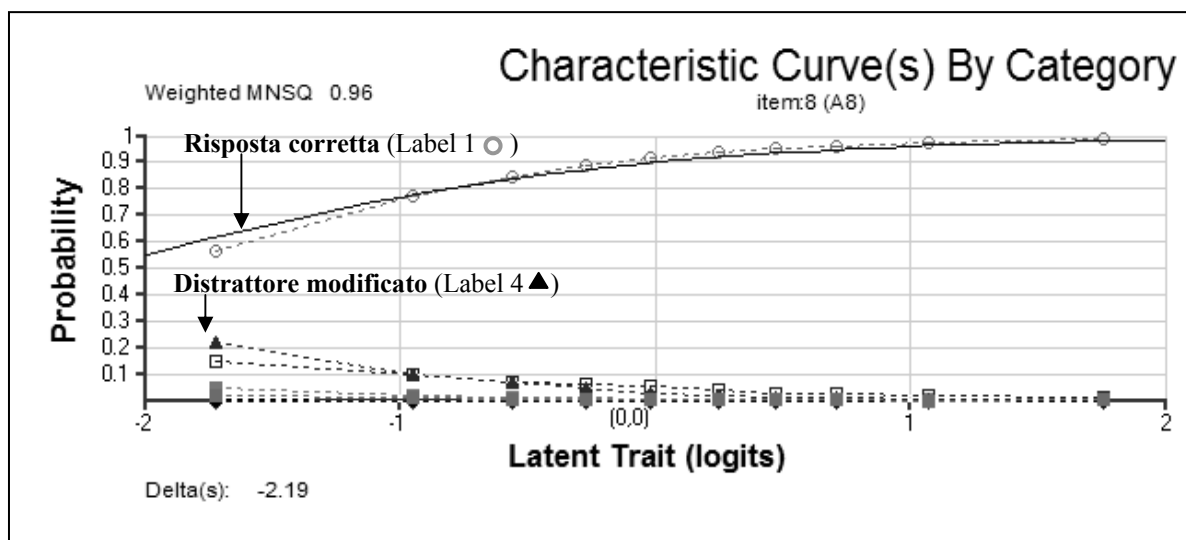
Figura 2.4: Curva caratteristica quesito A8
