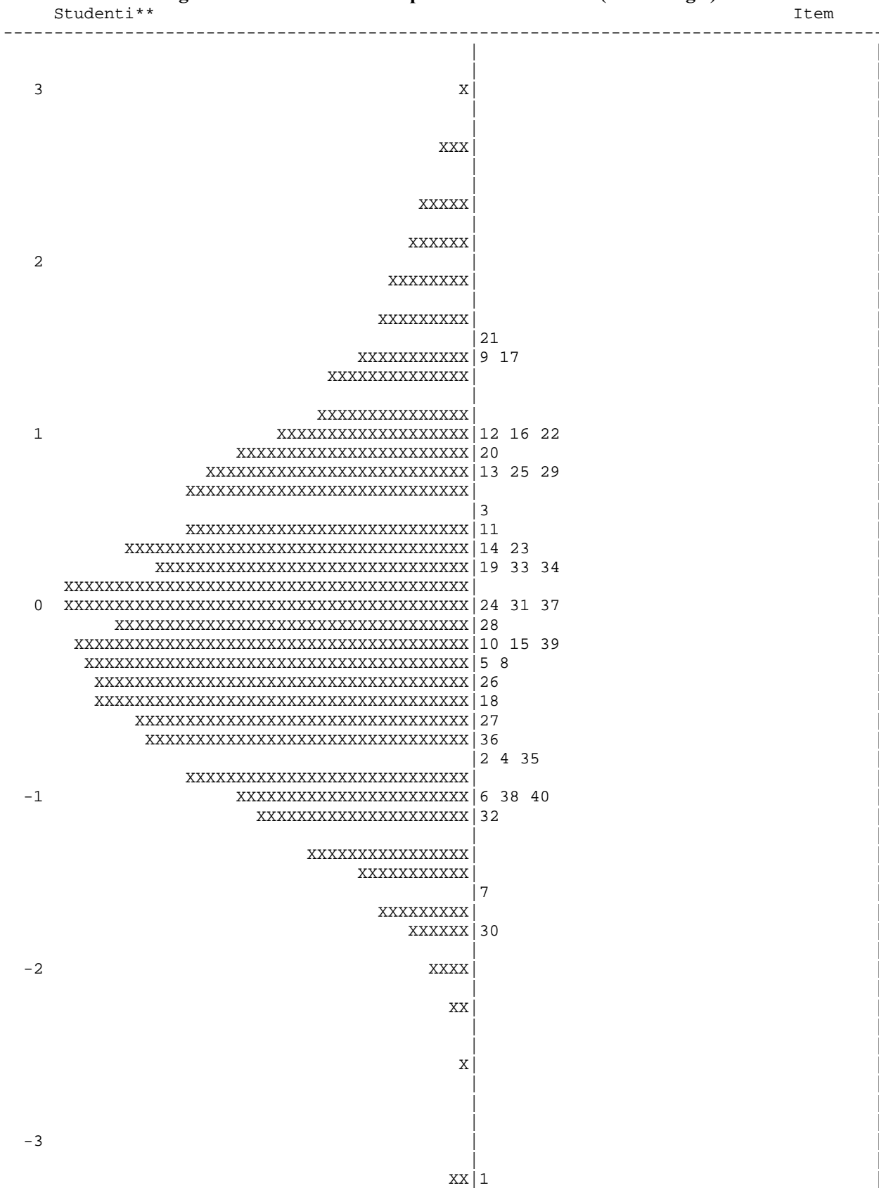
Figura 5.8: Placement della prova di Matematica (III sec. I gr.)*
