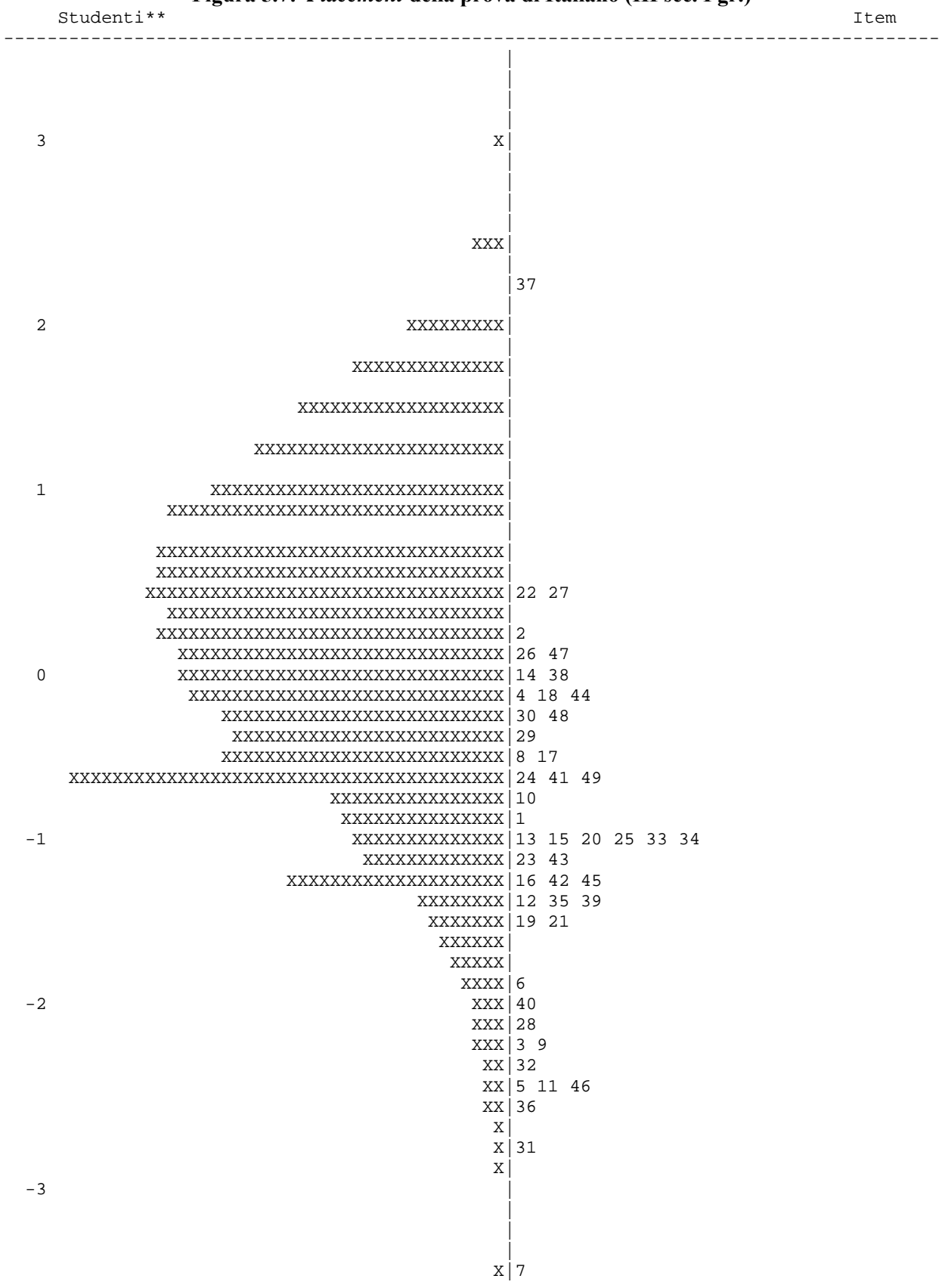
Figura 5.7: Placement della prova di Italiano (III sec. I gr.)*
