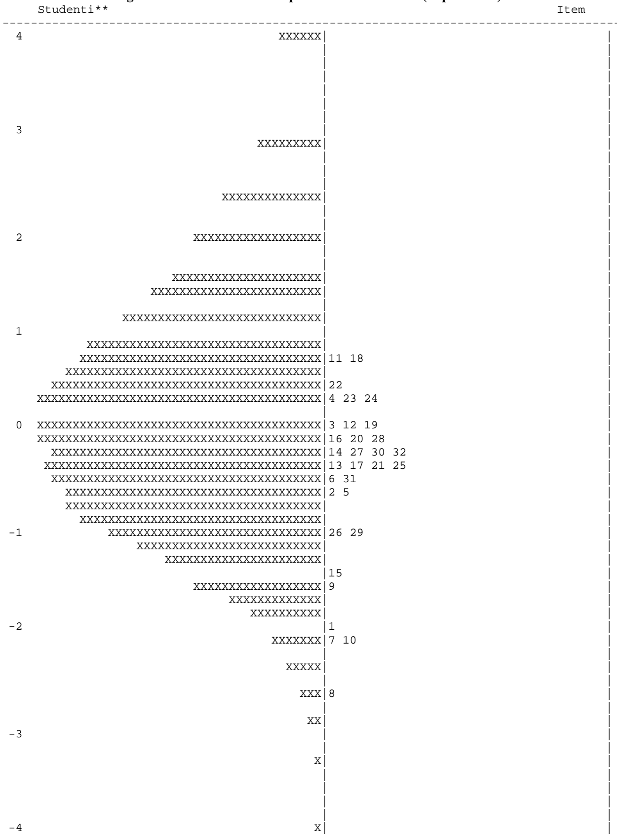
Figura 5.2: Placement della prova di Matematica (II primaria)*
