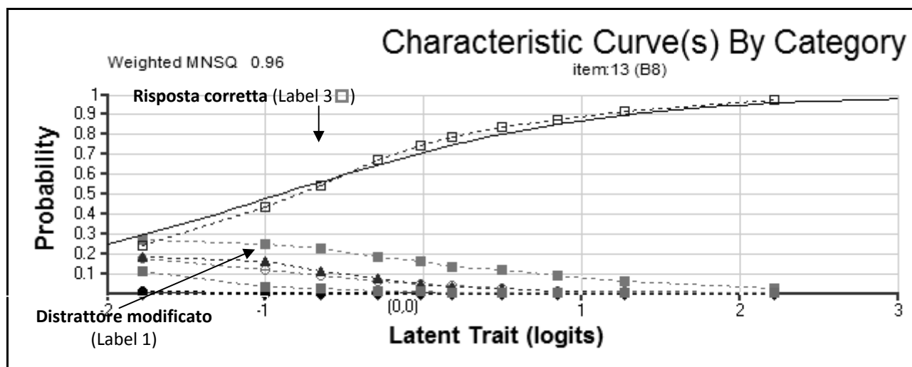
Figura 2.2: Curva caratteristica quesito B8
